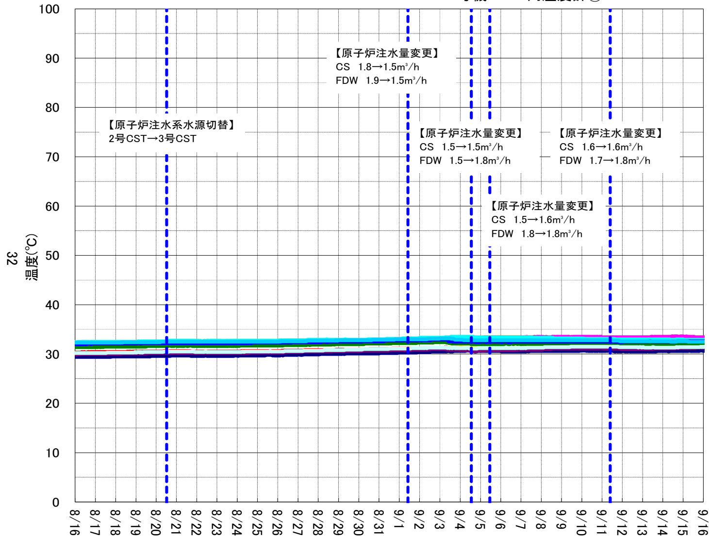
3号機 PCV内温度計①
