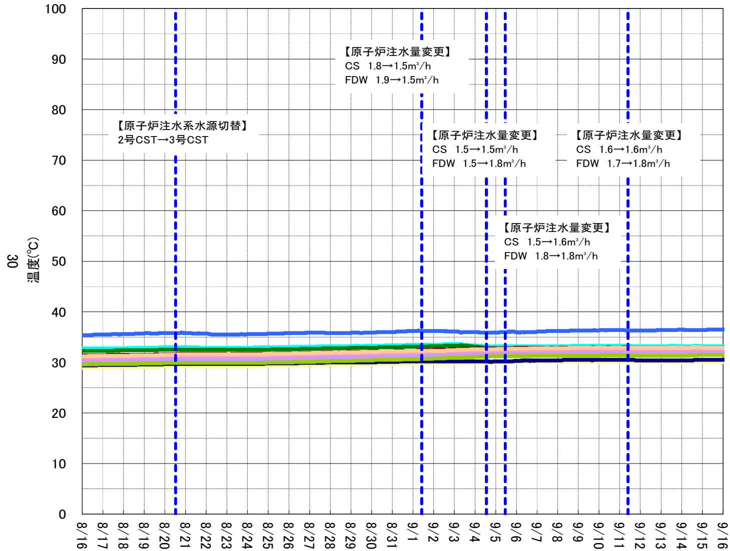
3号機 RPV周辺温度計(上部)
