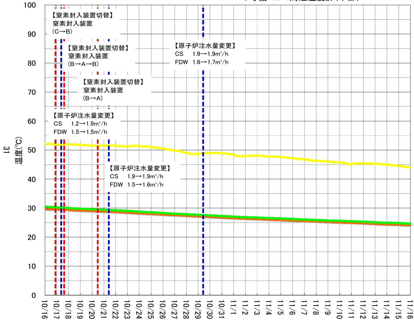
3号機 RPV周辺温度計(下部)
