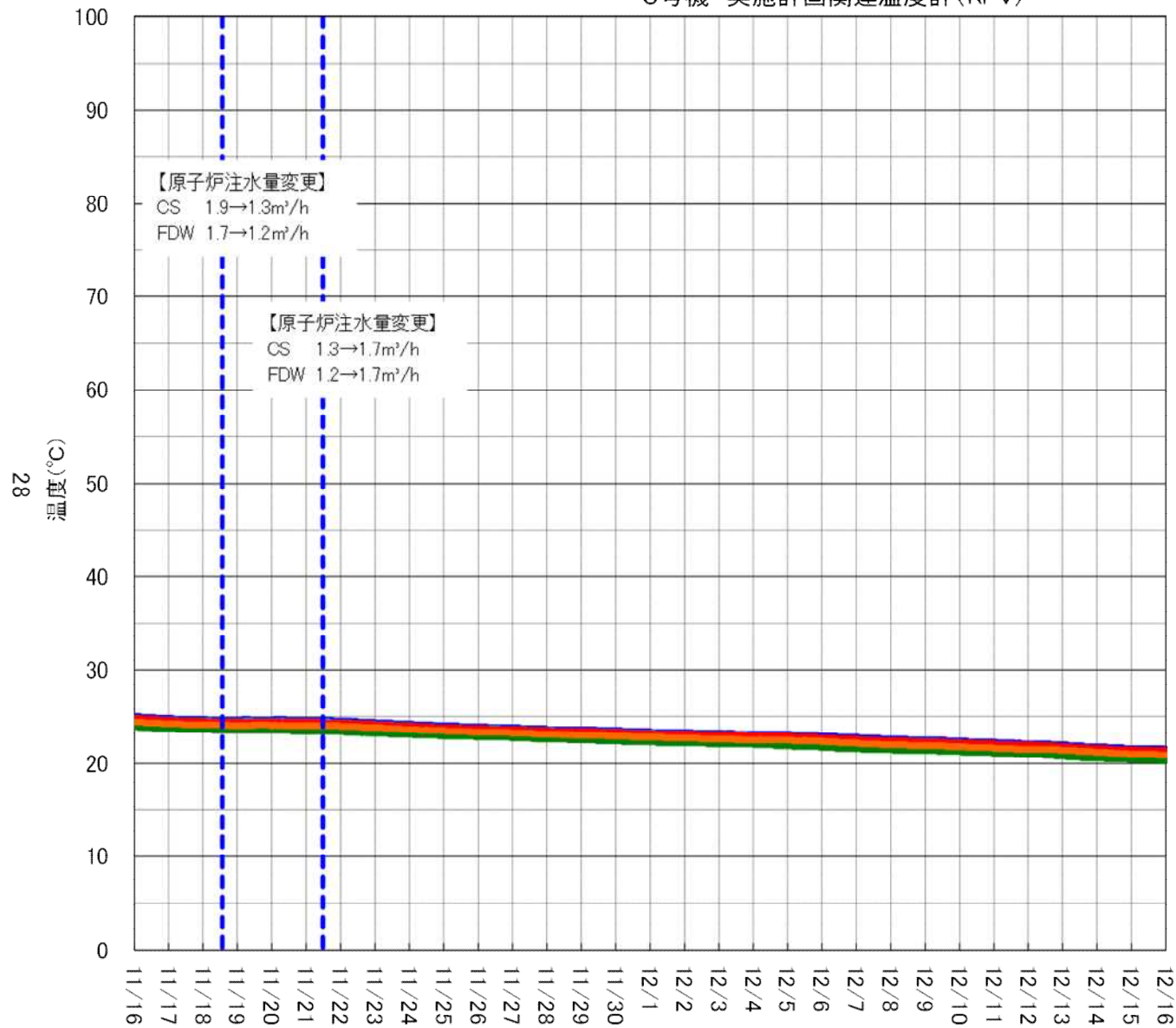
3号機 実施計画関連温度計(RPV)
