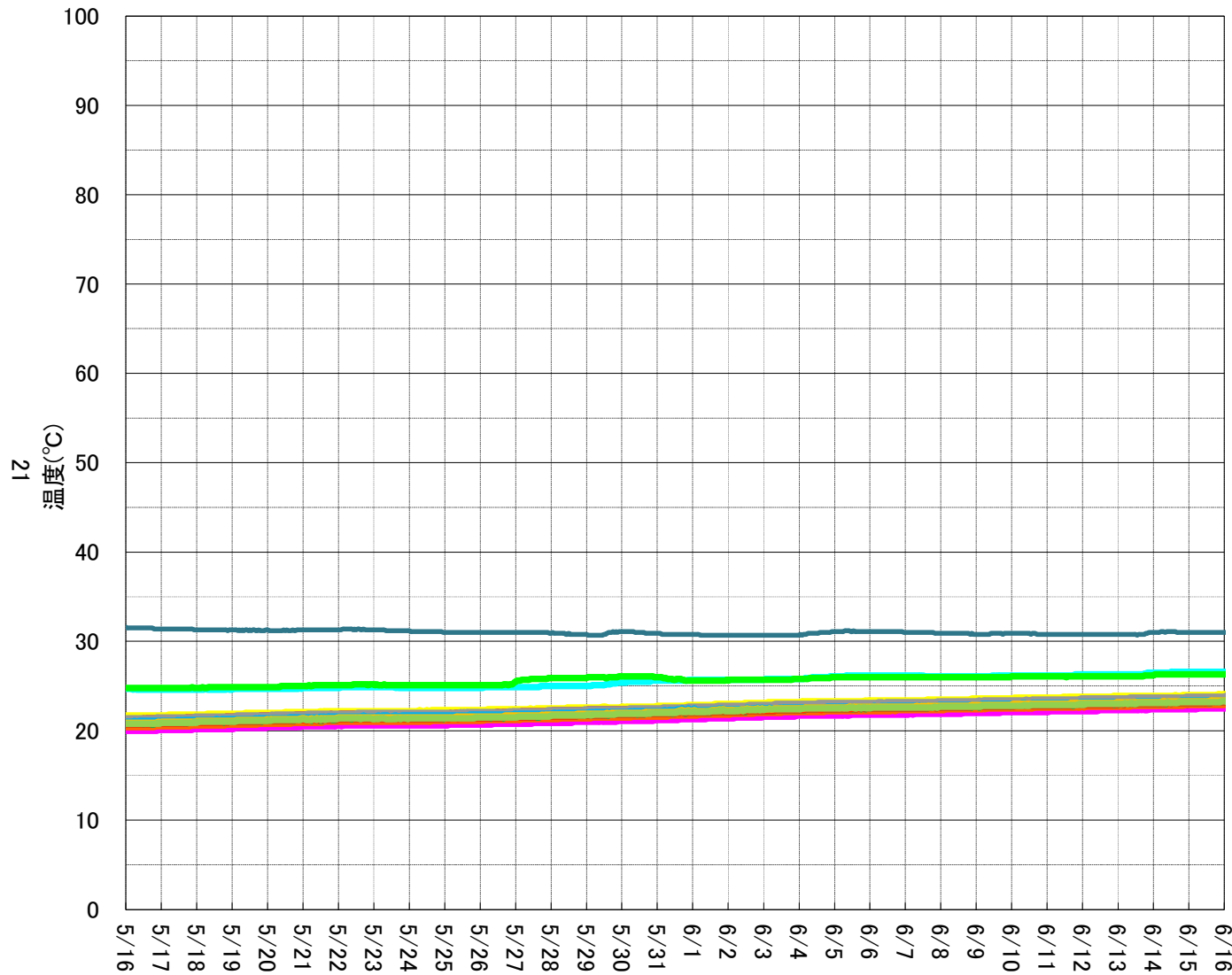
1号機 PCV内温度計
