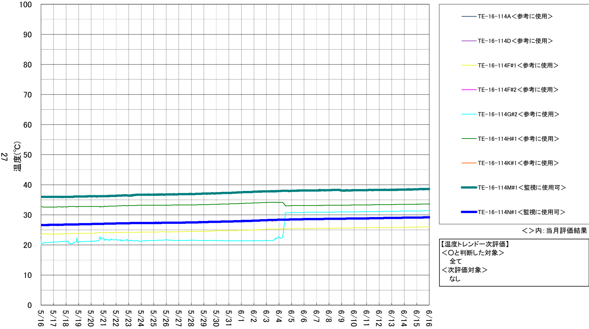
2号機 PCV内温度計②
