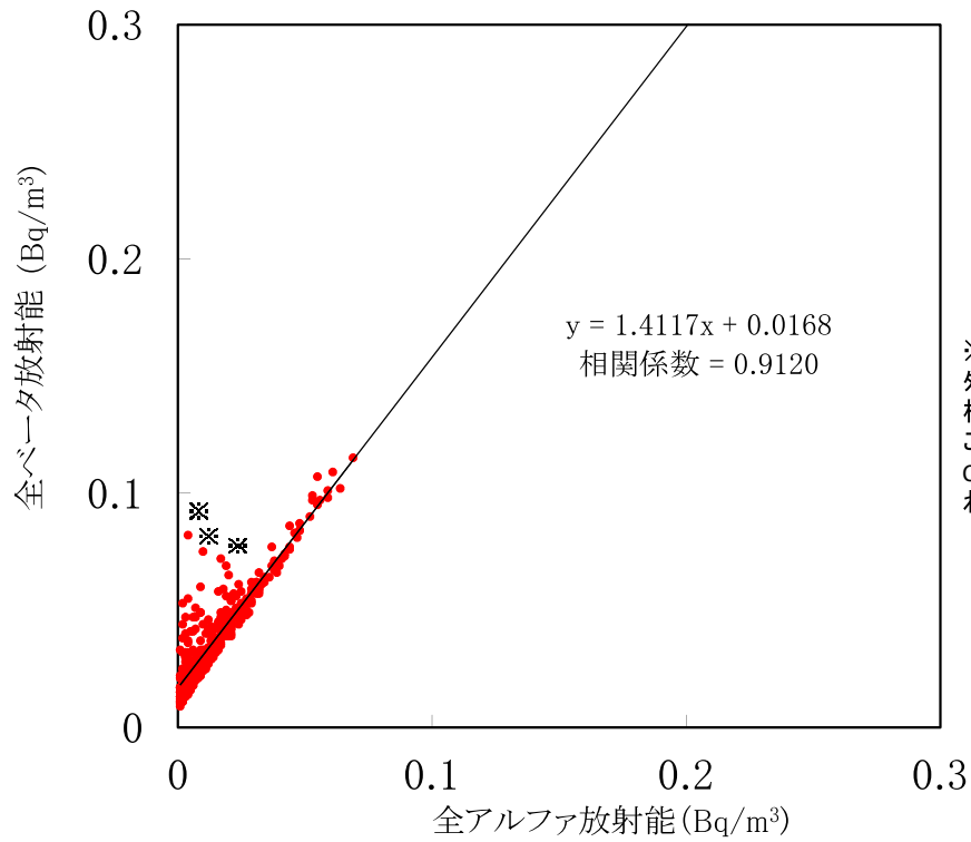
大気浮遊じんの全アルファ・全ベータ放射能の相関図 (MP-3) (令和7年10月～令和7年12月)
