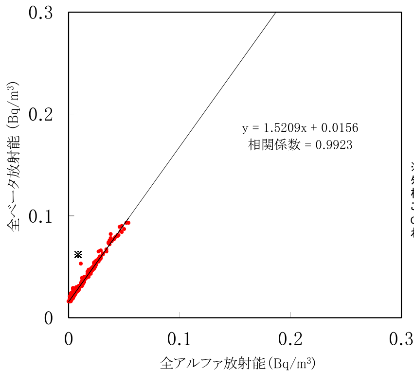
大気浮遊じんの全アルファ・全ベータ放射能の相関図 (MP-8) (令和7年10月～令和7年12月)
