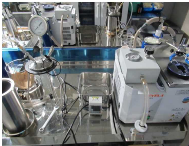
燃焼装置外観
