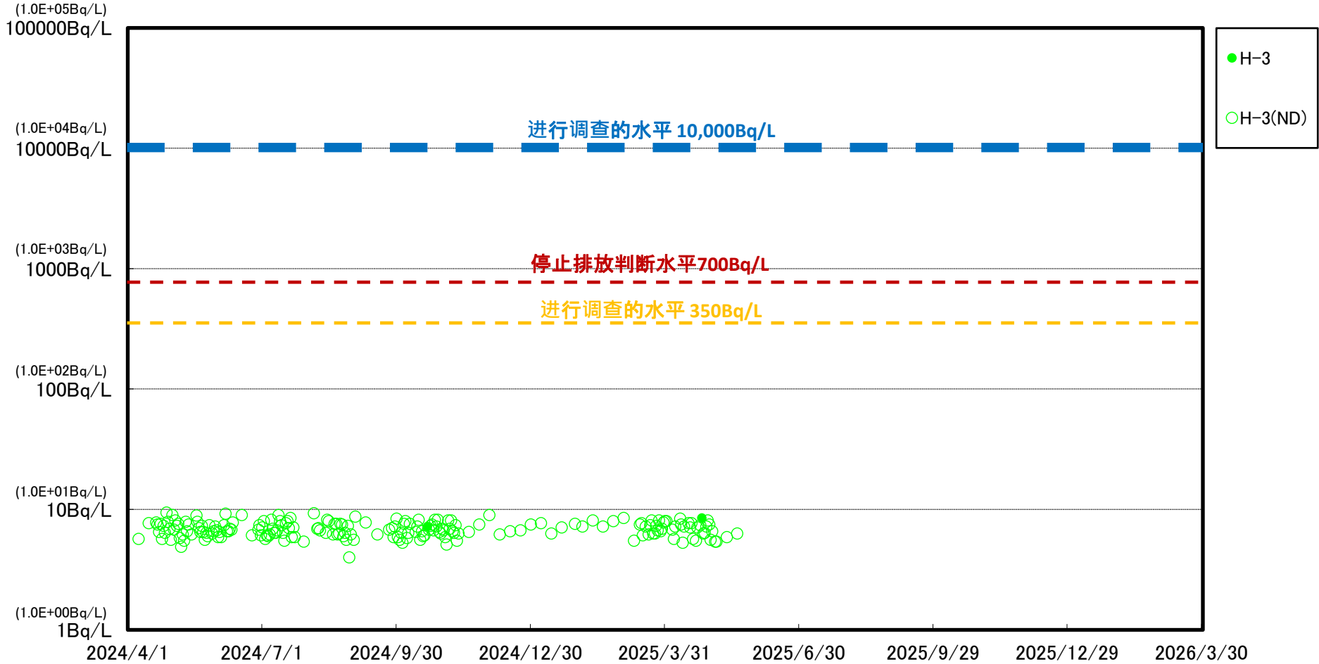
1F 北防波堤北側(T-0-1) 海水放射性浓度(可快速得出结果的测量)
