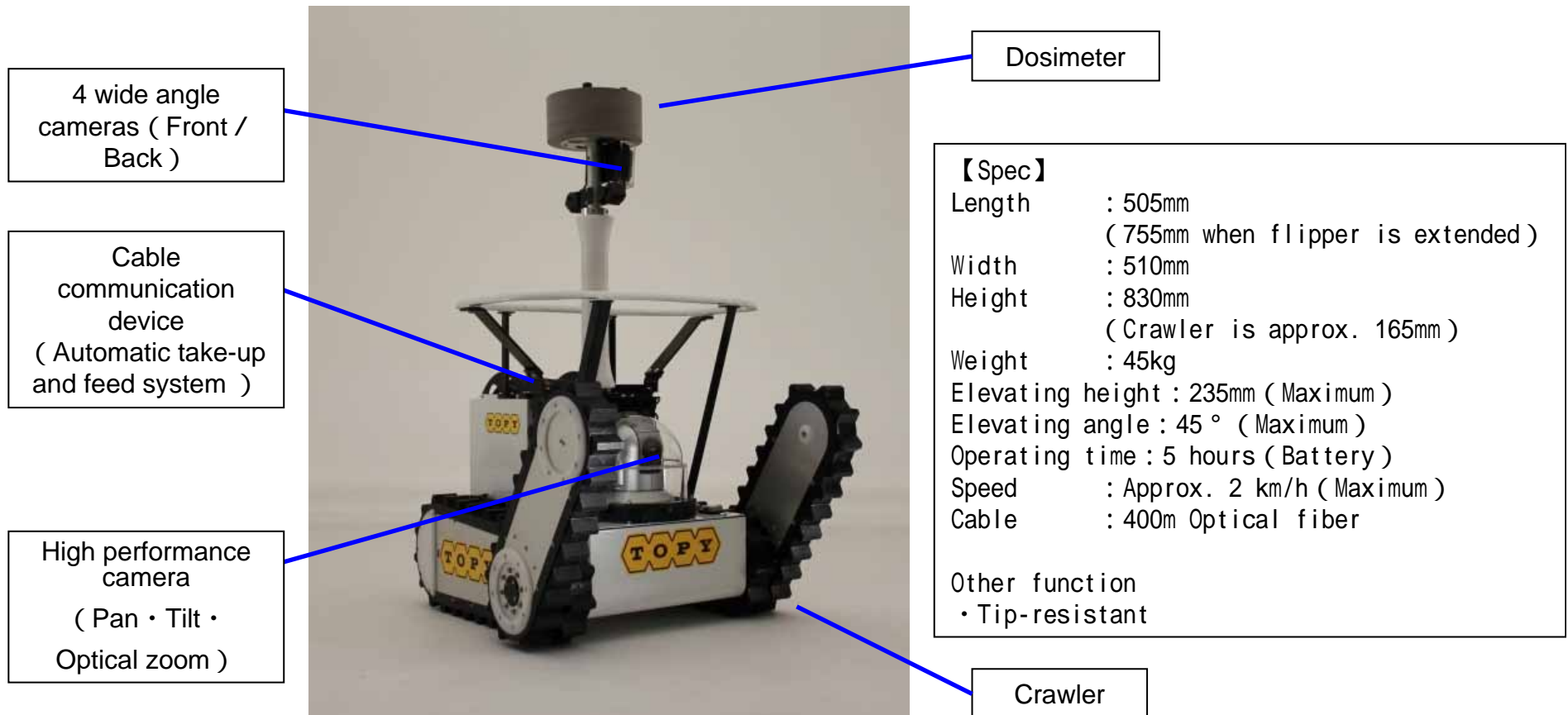
【Survey Runner, main body】
