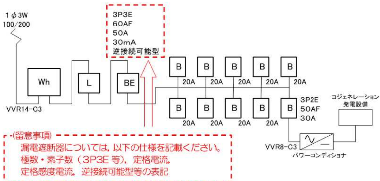
単線結線図（系統への逆潮流がない場合の例）
