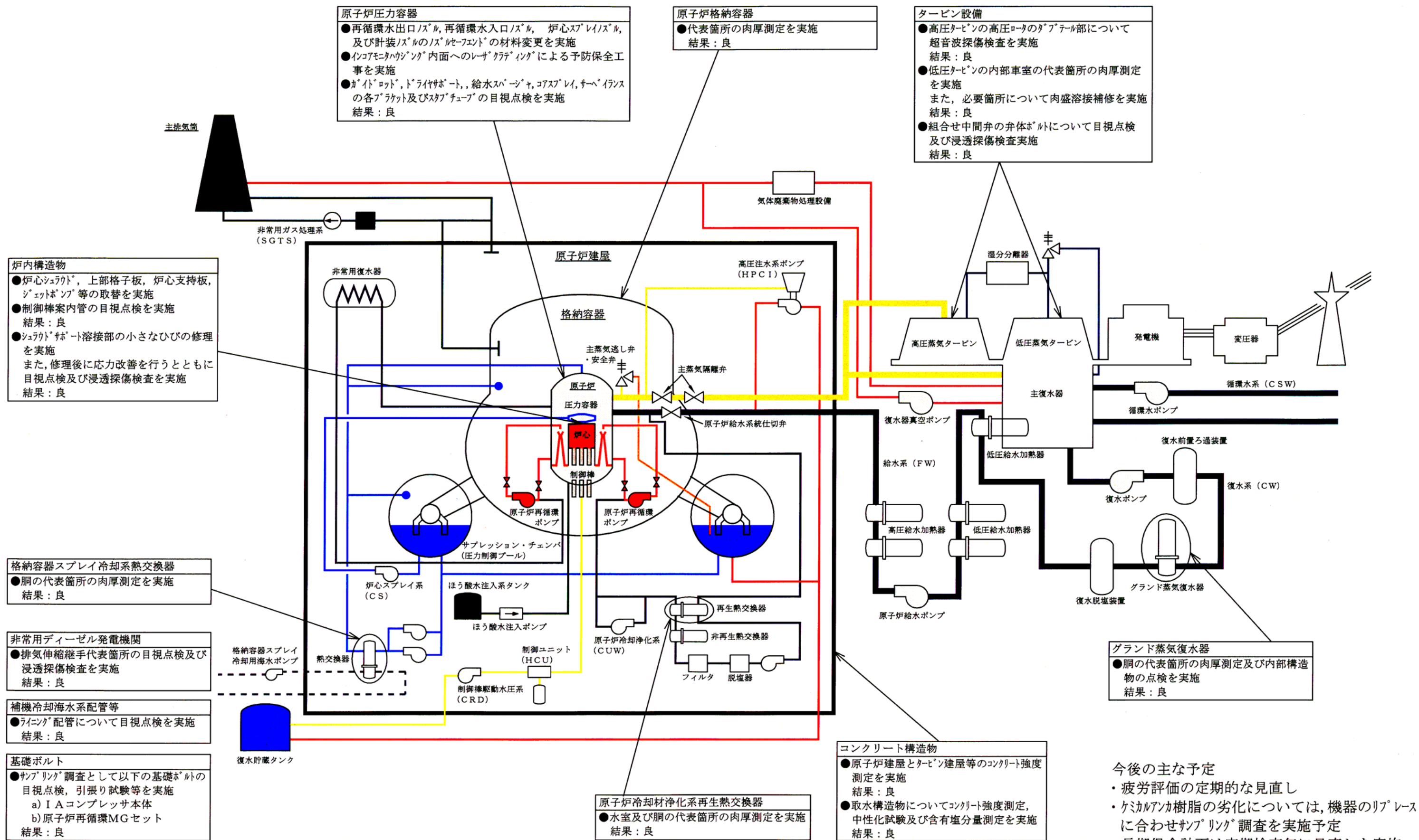
福島第一・1号機長期保全計画の実施状況
