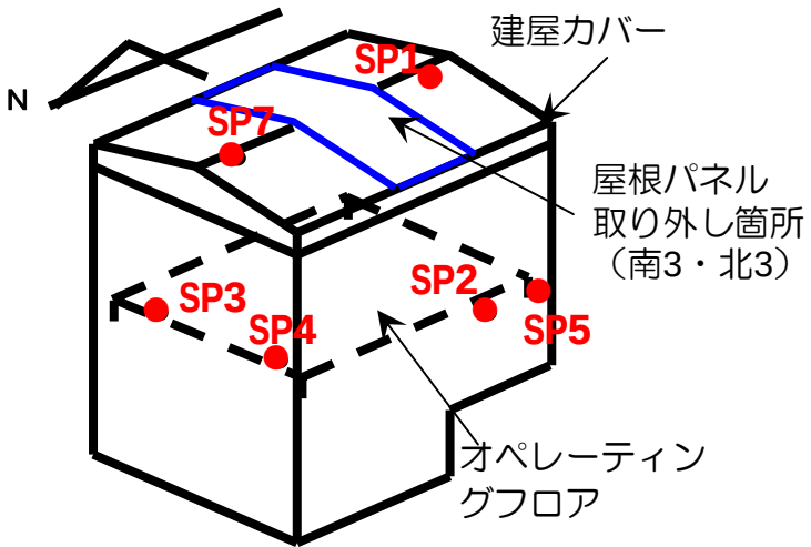
ダストモニタのサンプリング箇所
