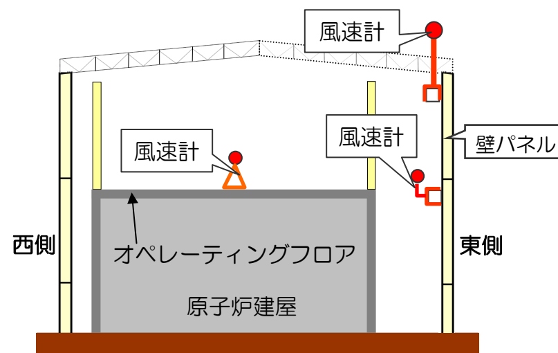
風速測定イメージ
