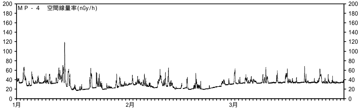
図2 MP - 4 ~ 6の空間線量率(低線量率) (測定期間:平成22年1月1日~平成22年3月31日)
