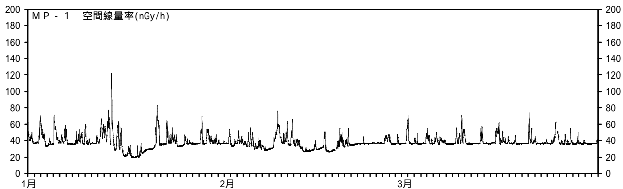
図1 MP - 1 ~ 3の空間線量率（低線量率） （測定期間：平成22年1月1日～平成22年3月31日）
