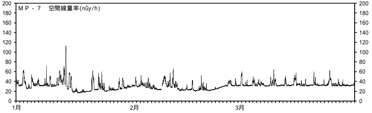
図3 MP - 7 ~ 9の空間線量率（低線量率） （測定期間：平成22年1月1日～平成22年3月31日）
