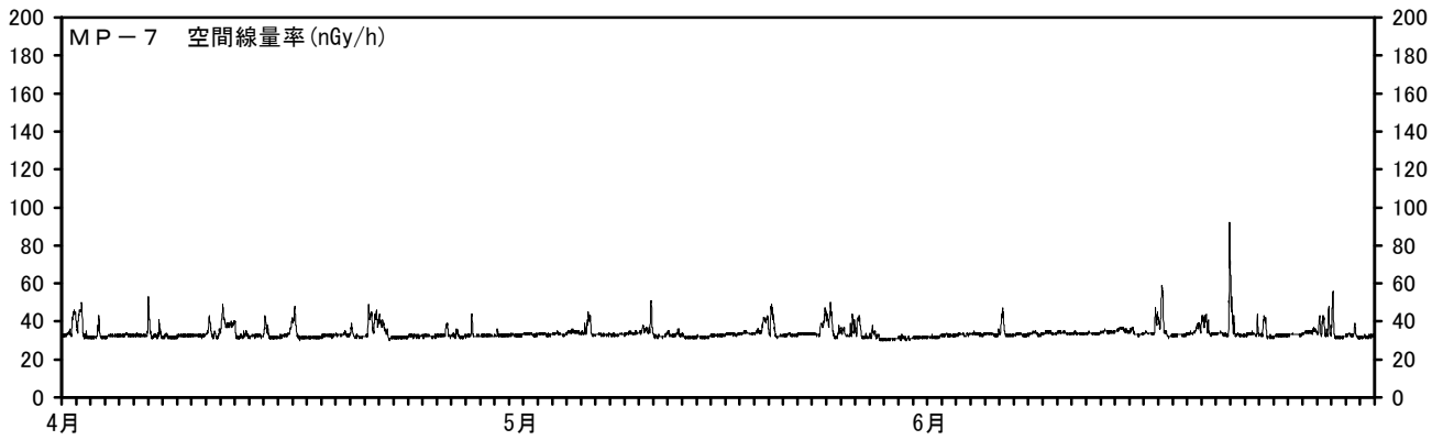
図3 MP-7～9の空間線量率（低線量率） （測定期間：平成22年4月1日～平成22年6月30日）
