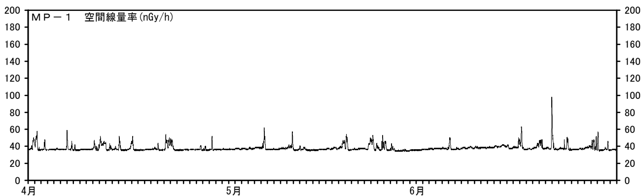
図1 MP-1～3の空間線量率（低線量率） （測定期間：平成22年4月1日～平成22年6月30日）
