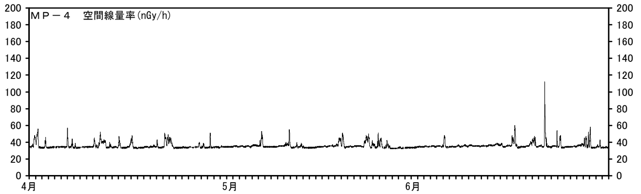
図2 MP-4～6の空間線量率（低線量率） （測定期間：平成22年4月1日～平成22年6月30日）
