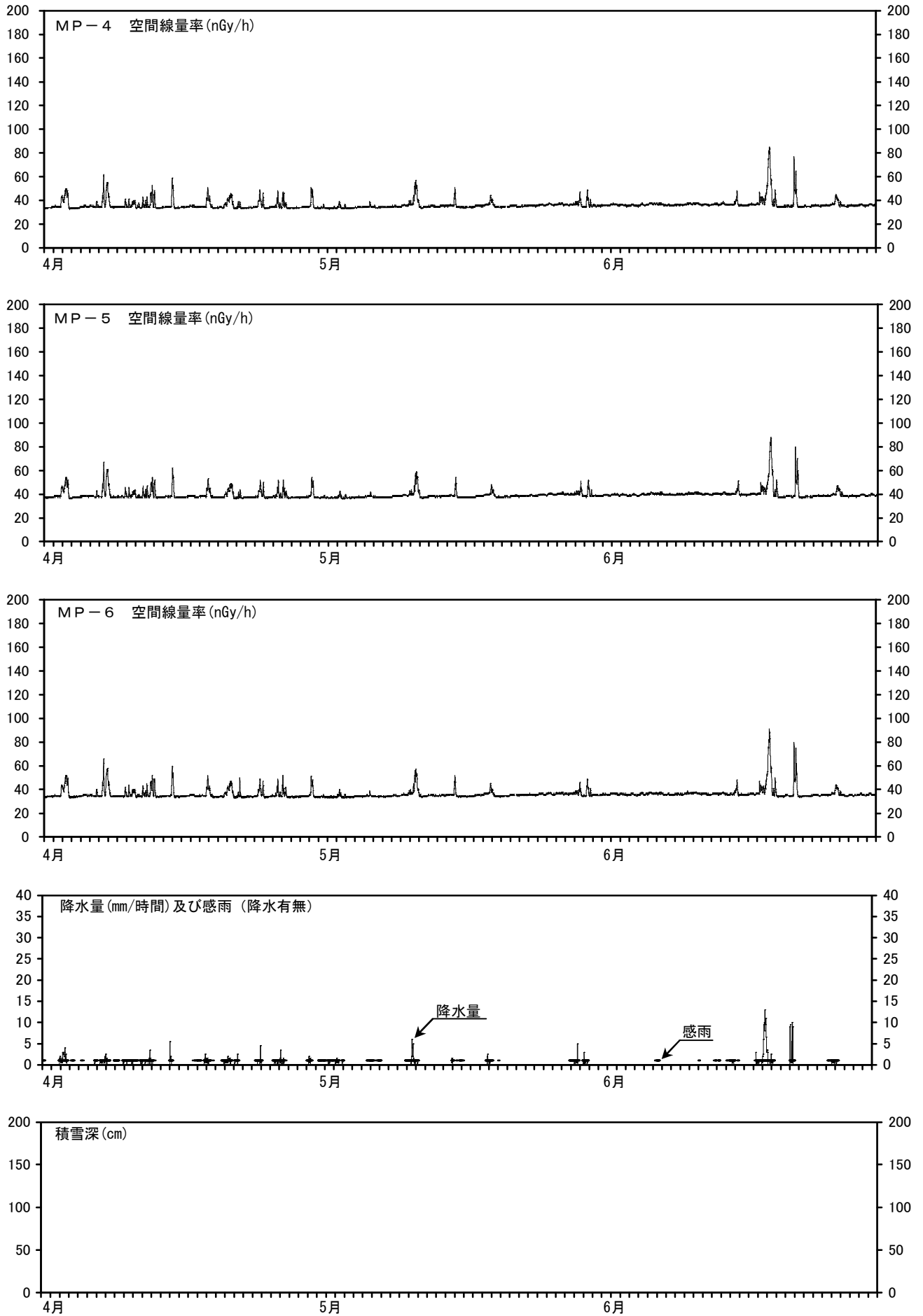
図2 MP-4～6の空間線量率（低線量率）と降水量及び積雪深との関係 (測定期間：平成25年4月1日～平成25年6月30日)
