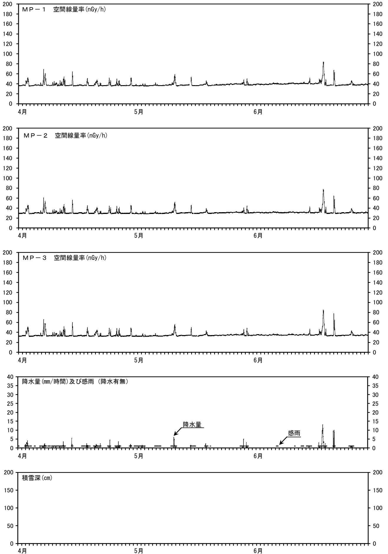
図1 MP-1～3の空間線量率（低線量率）と降水量及び積雪深との関係 （測定期間：平成25年4月1日～平成25年6月30日）
