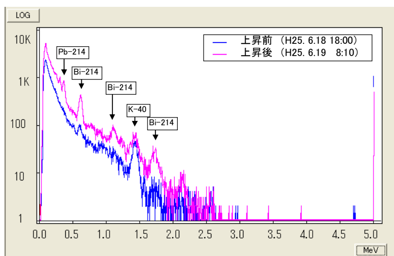
図2 スペクトル解析結果(MP-6 上昇前後)
