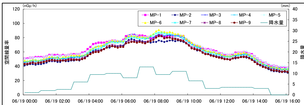
図1 空間線量率（10分値）及び降水量（1時間値）の推移
