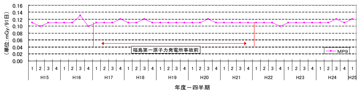
図 MP-9 地点における積算線量の推移（平成15年度以降）
