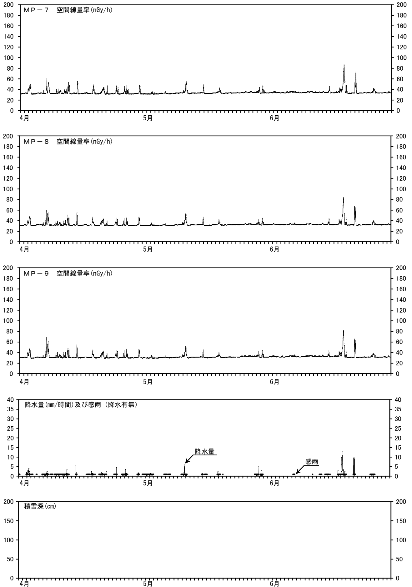
図3 MP-7～9の空間線量率（低線量率）と降水量及び積雪深との関係 （測定期間：平成25年4月1日～平成25年6月30日）
