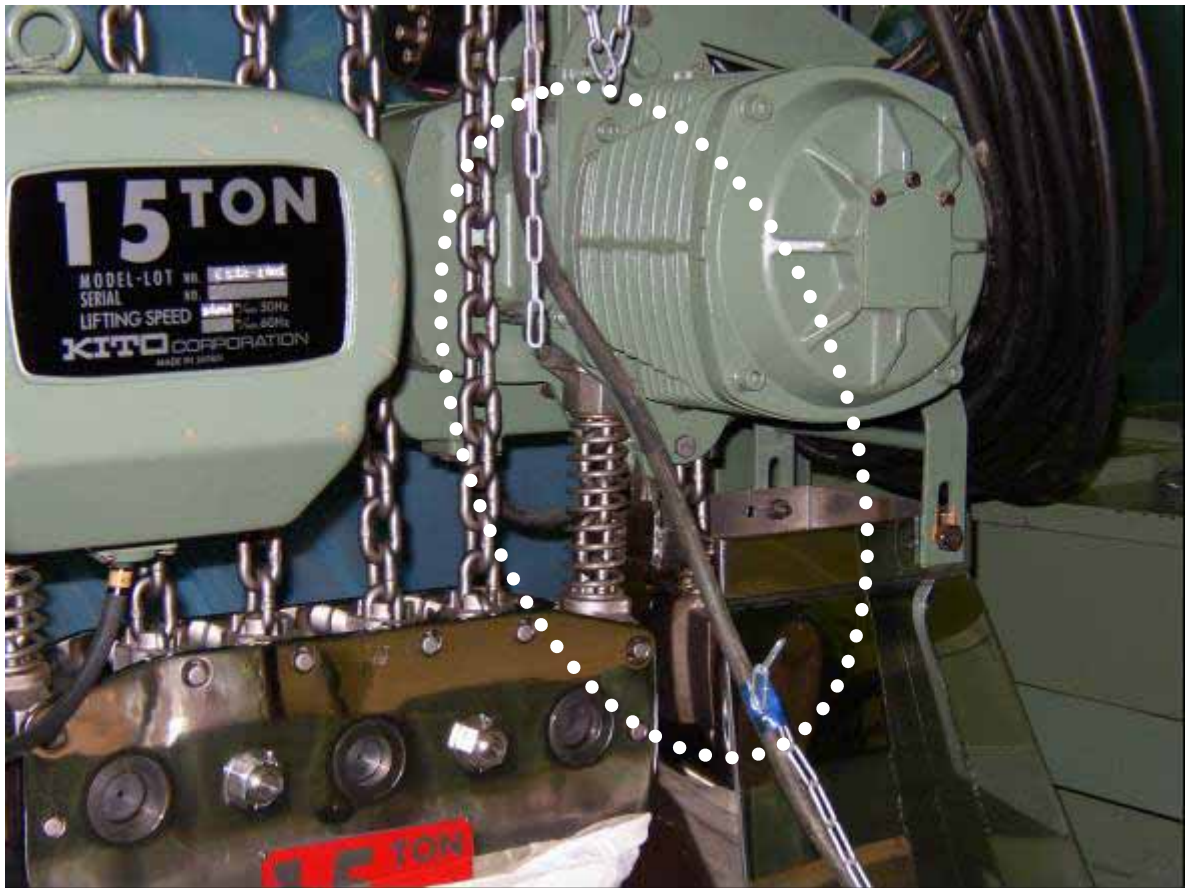
チェーン切断箇所の写真
