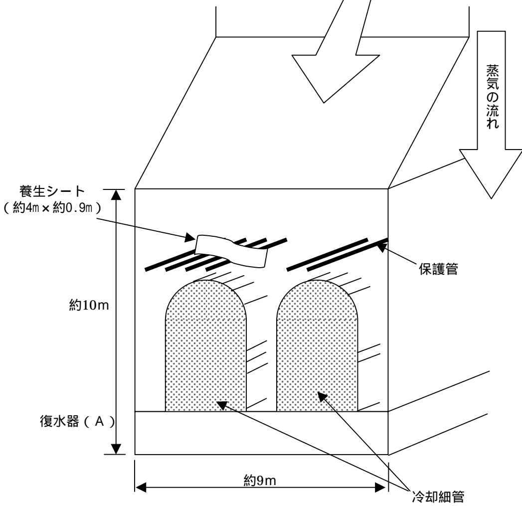
主復水器概略図
