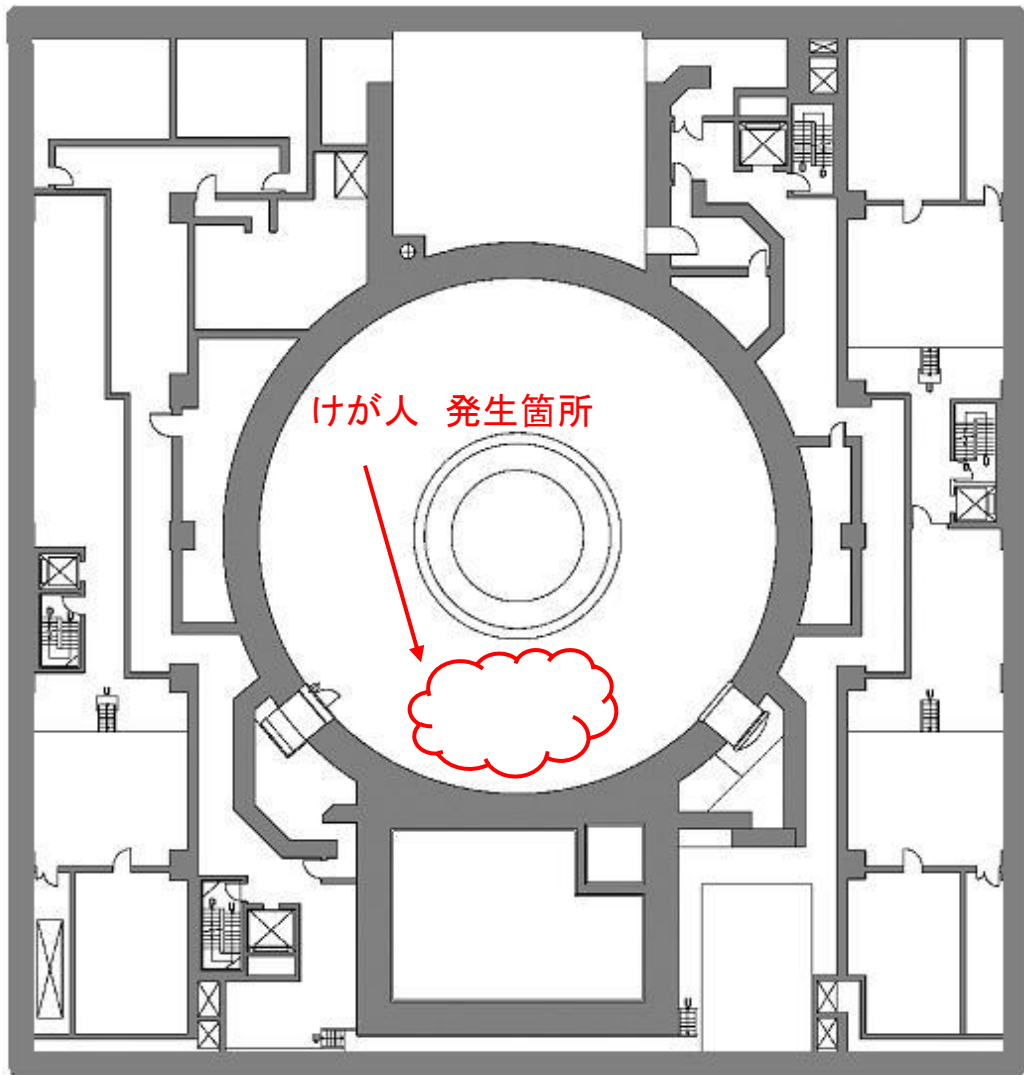
柏崎刈羽原子力発電所7号機 原子炉建屋 2階
