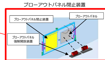
屋内外の設備・配管等の耐震工事 (屋内外複数箇所) ⇒2020年12月 工事完了
