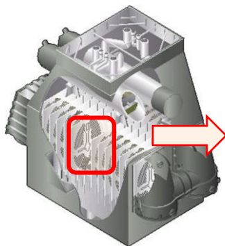
主復水器
