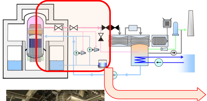
原子炉隔離時冷却系 (RCIC)
