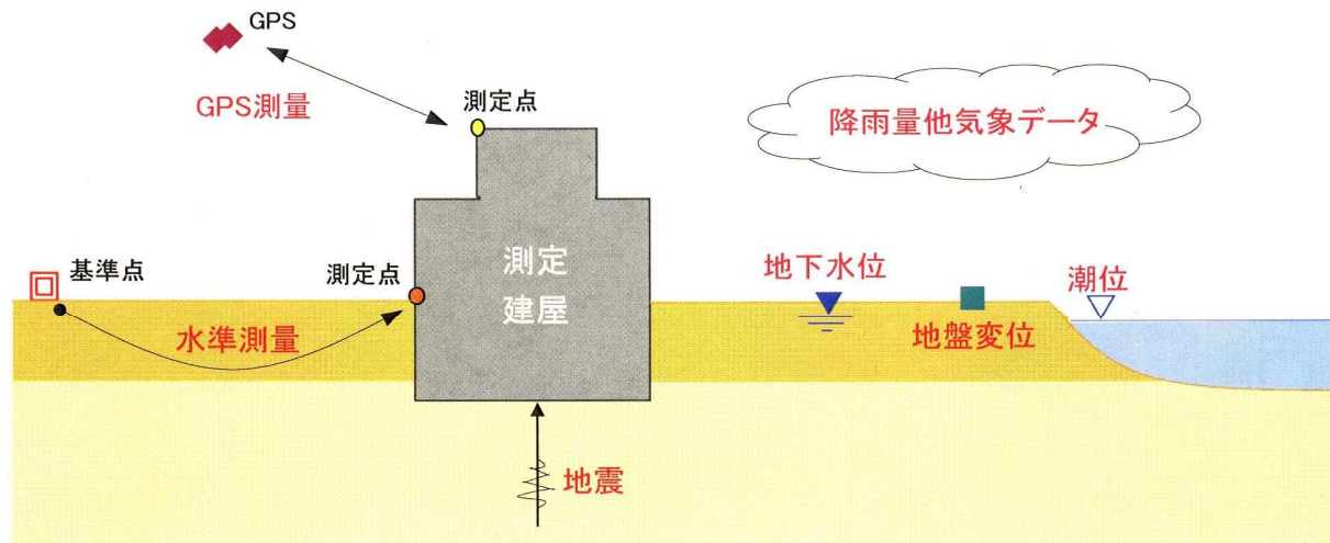
【測定概念図】
