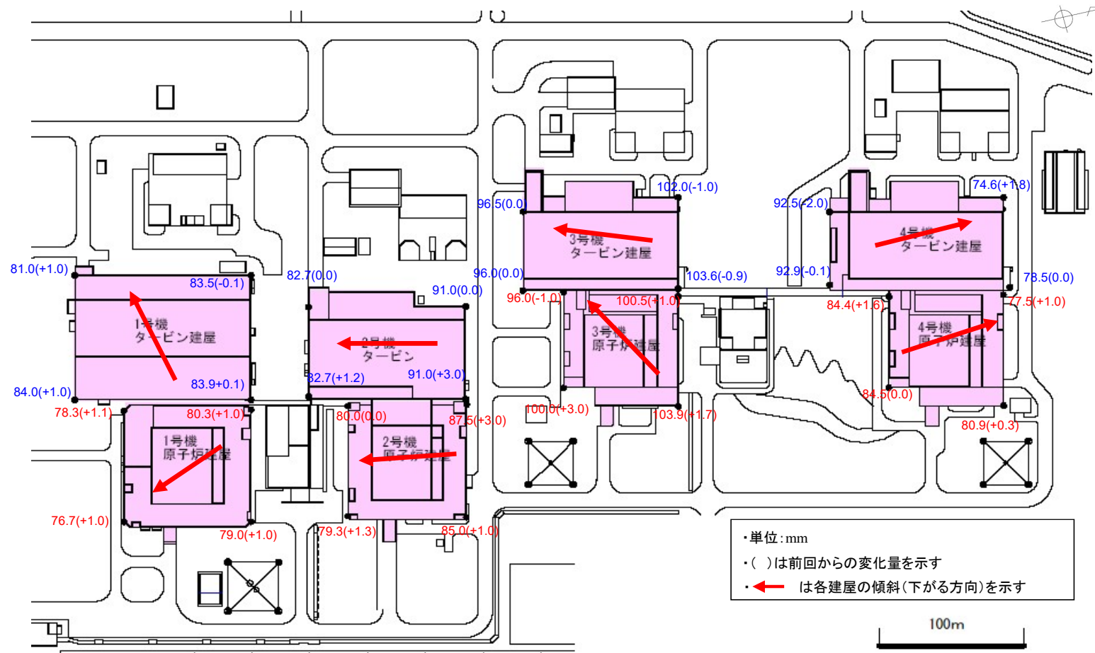
(1～4号機配置図)
