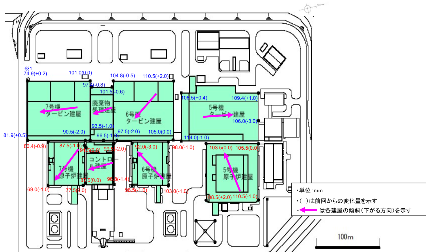
(5～7号機配置図)
