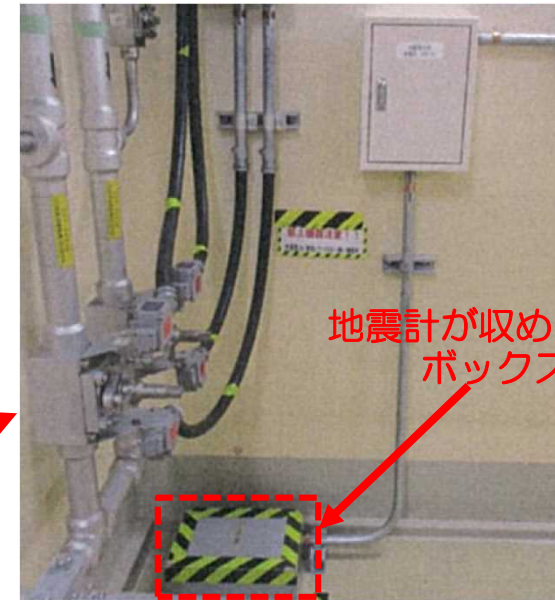
【地下5階（基礎版）での設置例】
