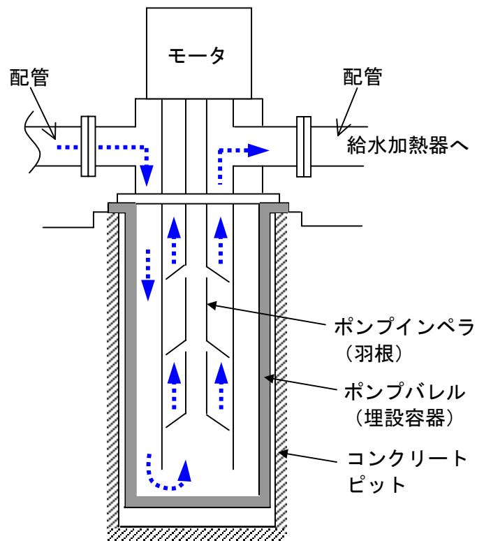
給水加熱器ドレンポンプ断面図
