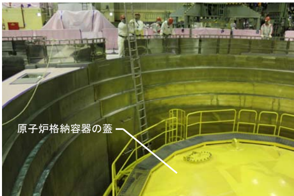
コンクリートハッチ 取り外し後の様子 (平成24年9月10日撮影)
