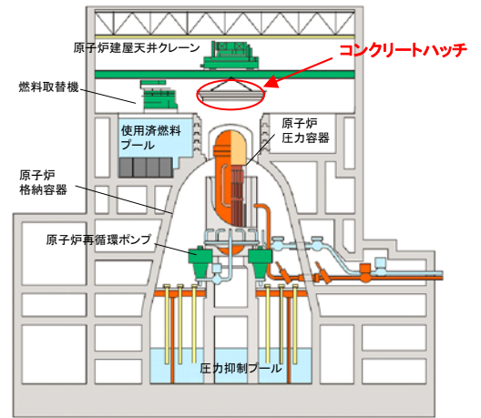
原子炉建屋 概略断面図 (コンクリートハッチ取り外し作業)
