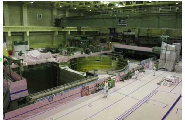
コンクリートハッチ 取り外し後の様子 (平成24年9月10日撮影)
