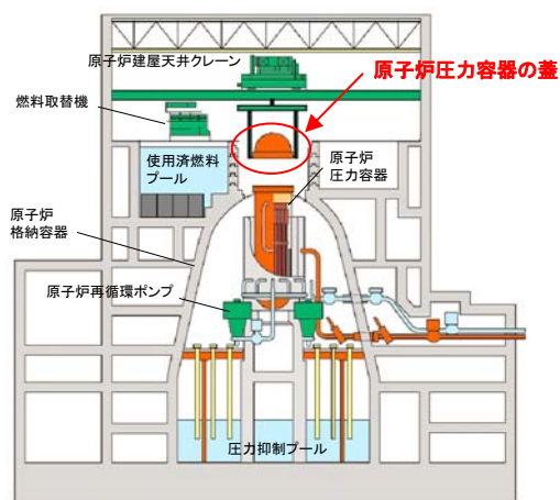
原子炉建屋 概略断面図 (原子炉圧力容器 蓋の取り外し作業)
