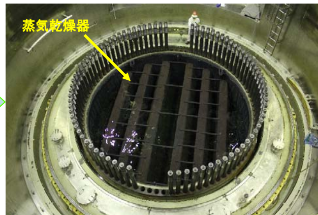
原子炉圧力容器 蓋の取り外し後の様子 (平成24年9月14日撮影)
