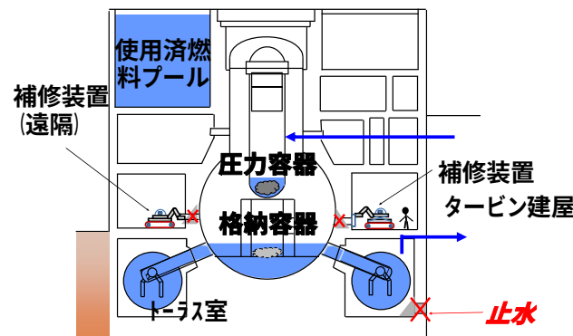
b) 建屋間、格納容器補修・止水 燃料デブリ取り出し作業（イメージ）
