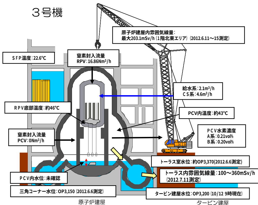
3号トーラス・階段室水位測定
