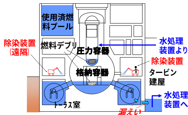
a) 原子炉建屋内除染
