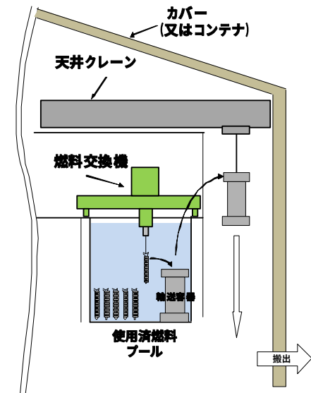
取り出し作業
