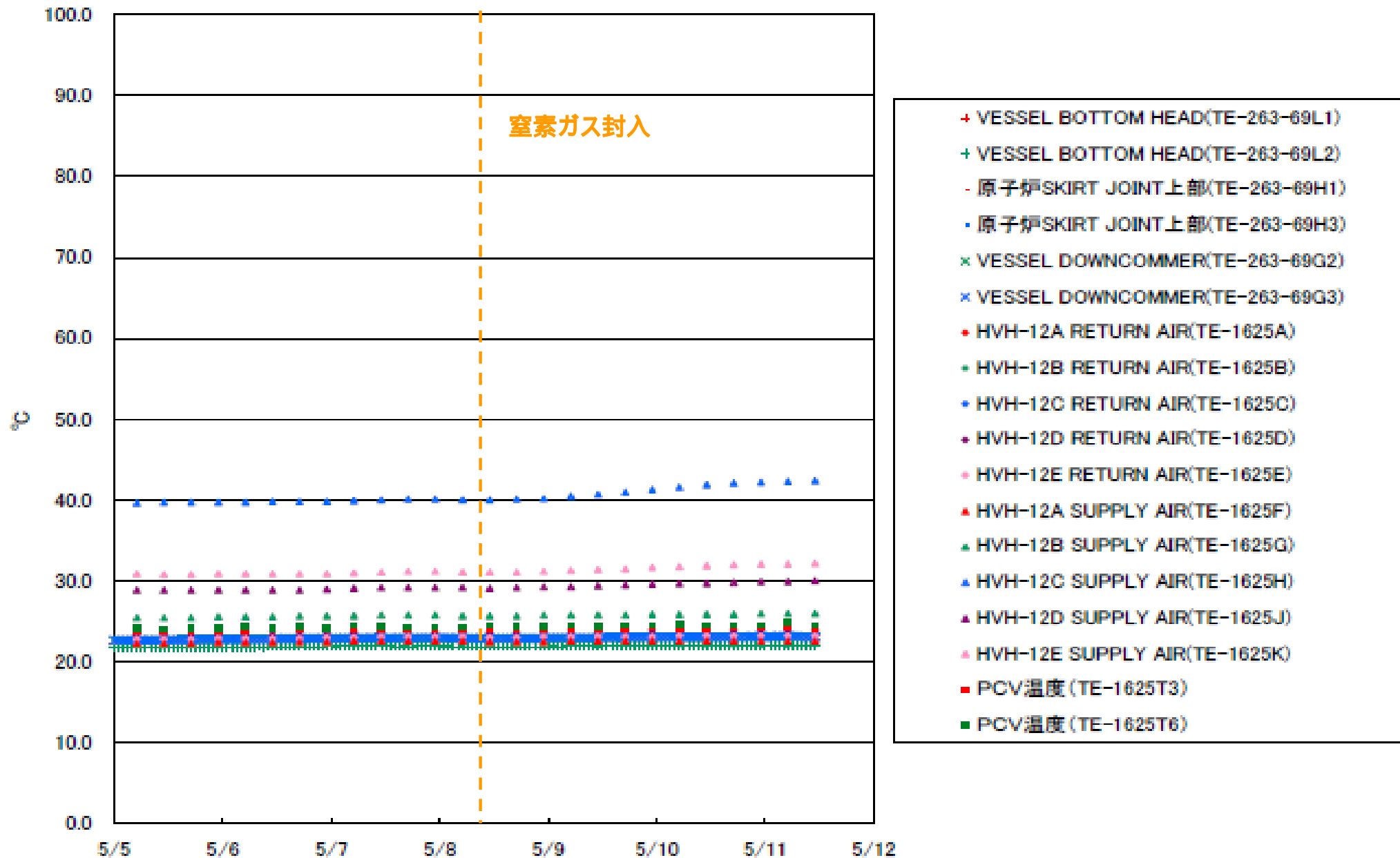
福島第一原子力発電所1号機 温度に関するパラメータ
