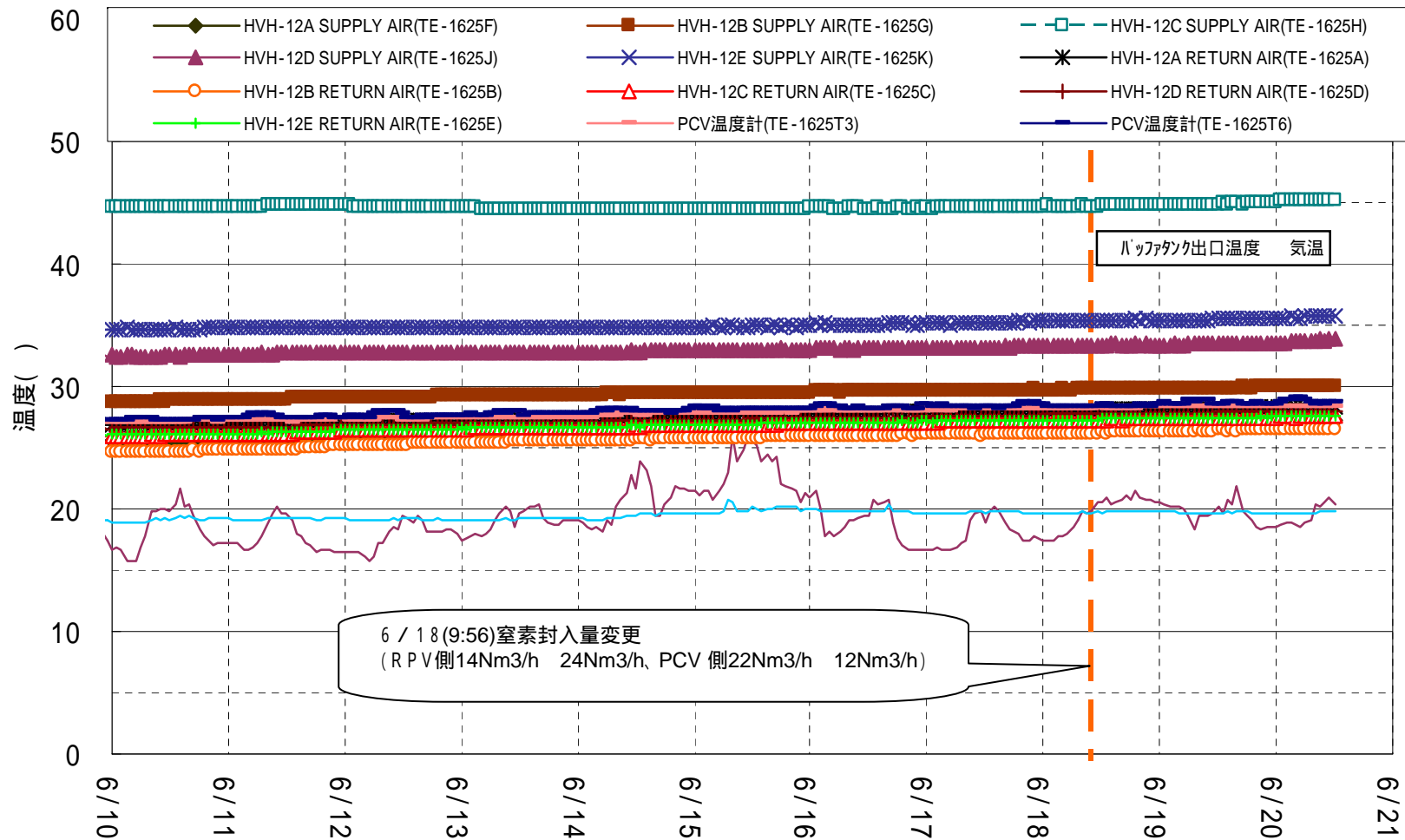
1号機原子炉格納容器内温度グラフ
