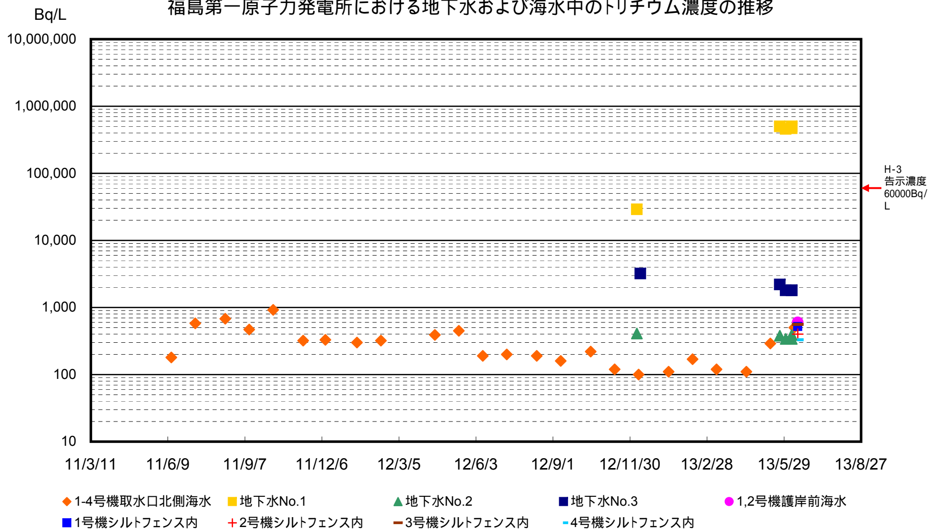
福島第一原子力発電所における地下水および海水中のトリチウム濃度の推移
