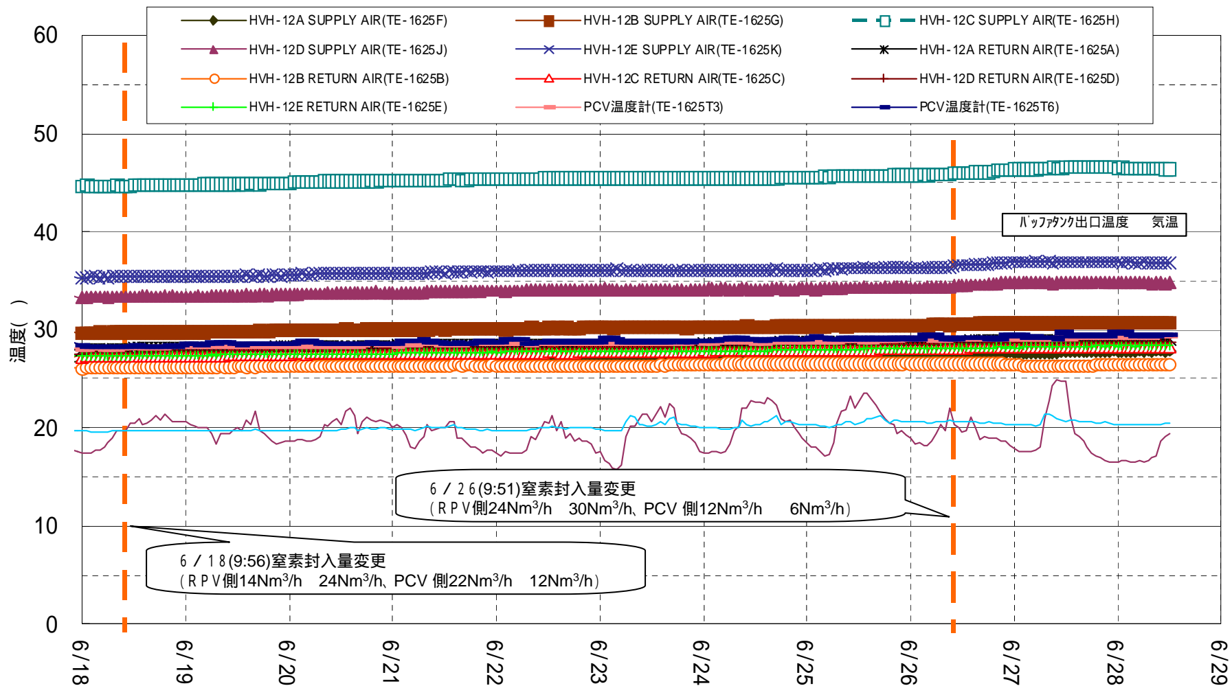
1号機原子炉格納容器内温度グラフ
