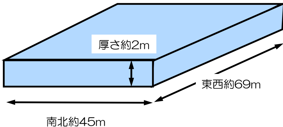
基礎概形イメージ図
