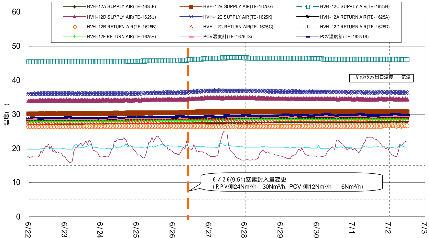
1号機原子炉格納容器内温度グラフ 流量変更時の計器指示値は約11.7Nm 3 /h
