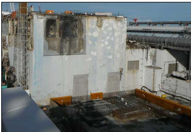
①鉄骨建方着手前 (平成24年12月18日)
