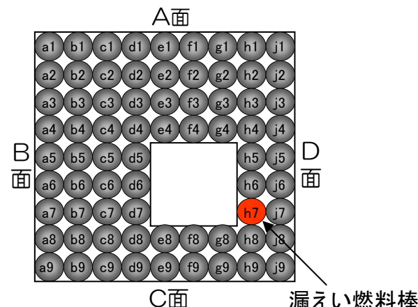
燃料集合体断面(F4UN22)
