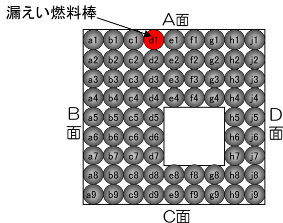
燃料集合体断面(F4UN4)
