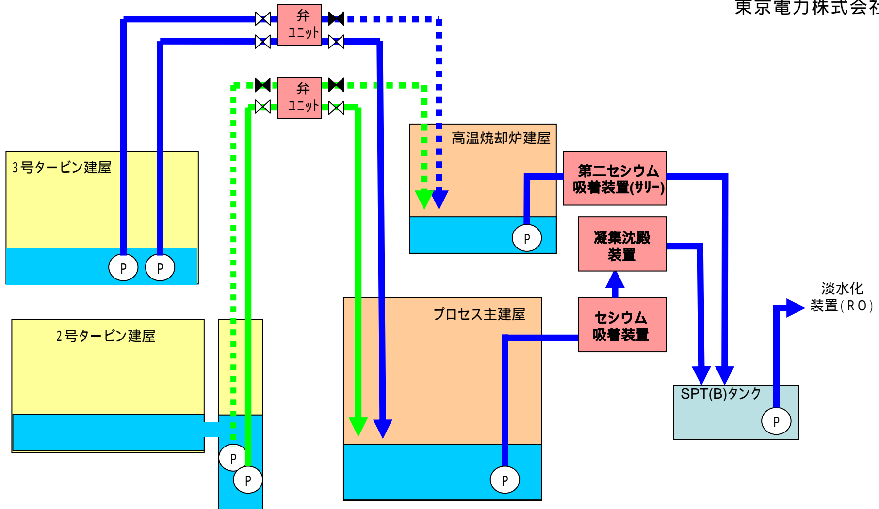
2 / 3号機タービン建屋滞留水の移送概念図
