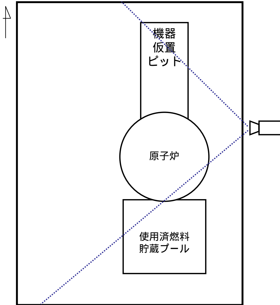
福島第一原子力発電所 2号機原子炉建屋 5階配置図
