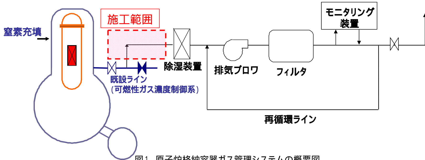
図1 原子炉格納容器ガス管理システムの概要図
