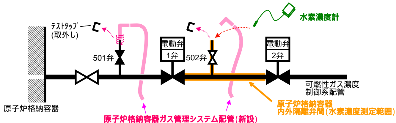
図2 ホース接続箇所及び水素ガス濃度測定箇所の拡大図
