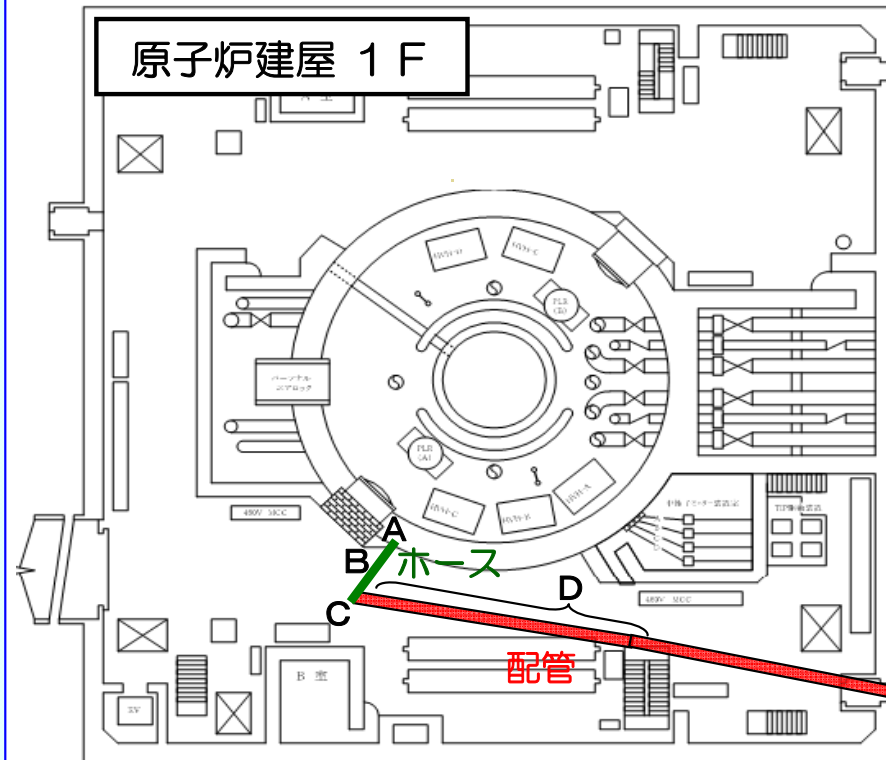
D. 配管部
