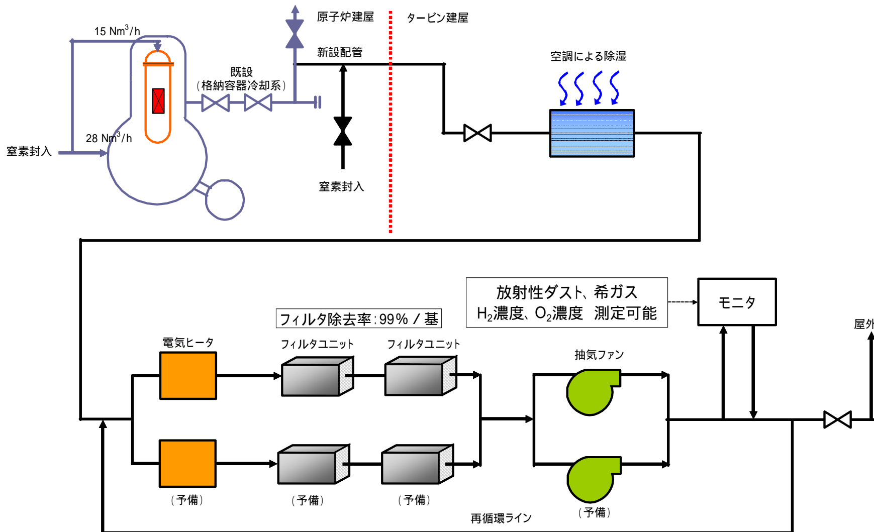
【系統構成概略図】
