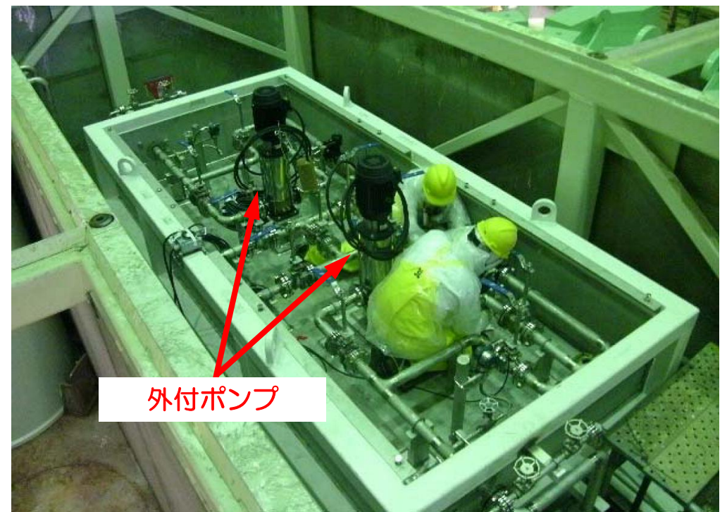
②セシウム吸着装置（ポンプスキッド） （平成24年5月31日 当社社員撮影）
