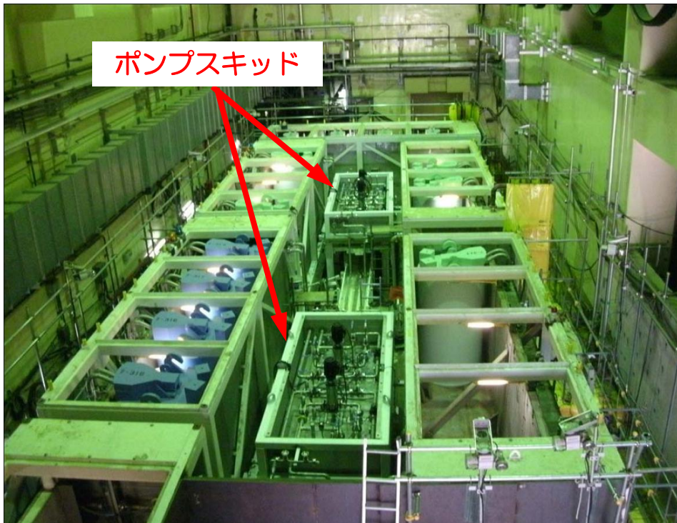
①セシウム吸着装置（全体） （平成24年6月4日 当社社員撮影）
