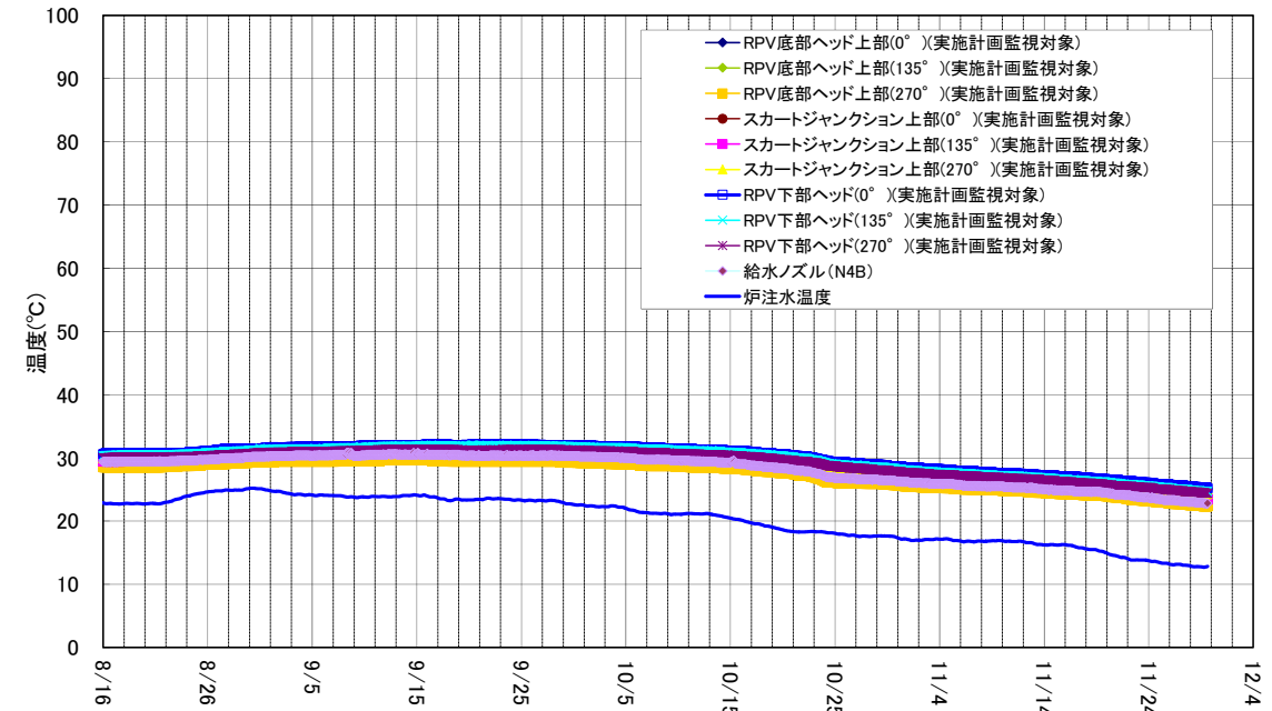
3号機 原子炉圧力容器まわり温度(8/16~11/29)
