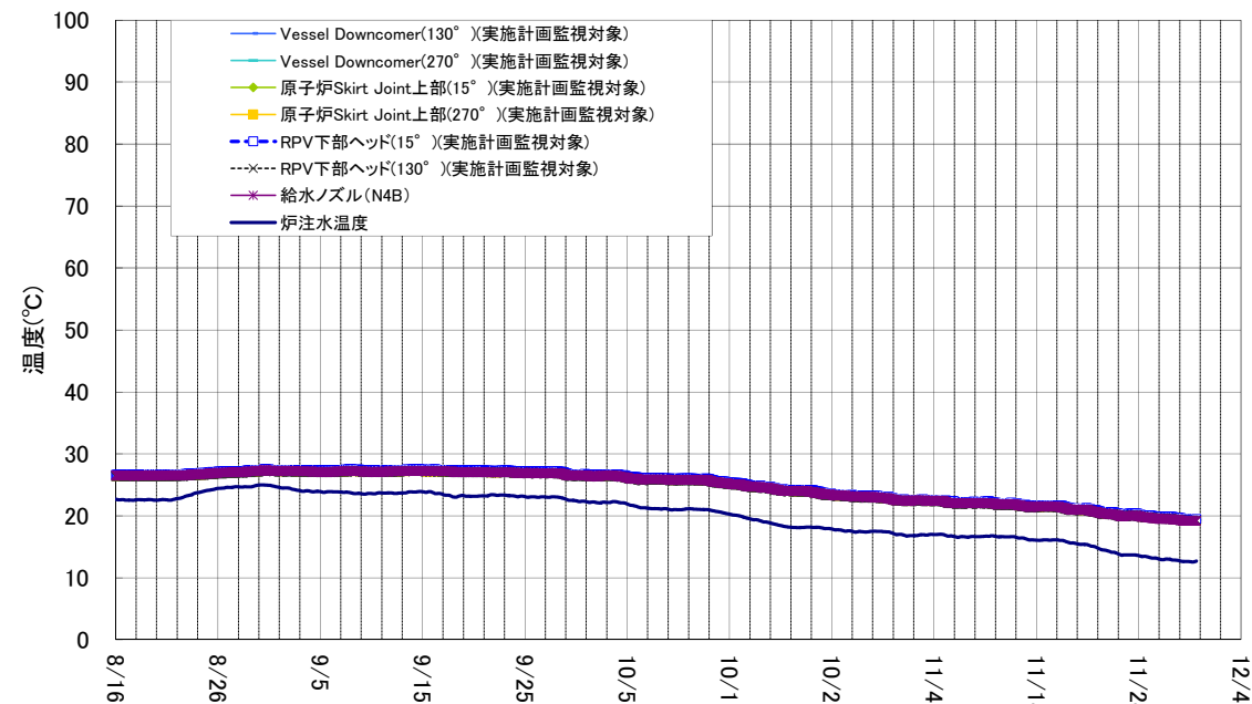
1号機 原子炉圧力容器まわり温度(8/16~11/29)
