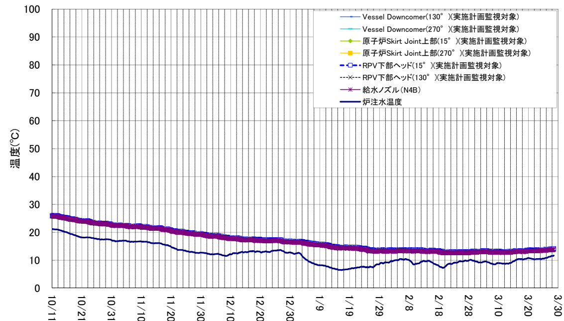
1号機 原子炉圧力容器まわり温度(10/11~3/28)
