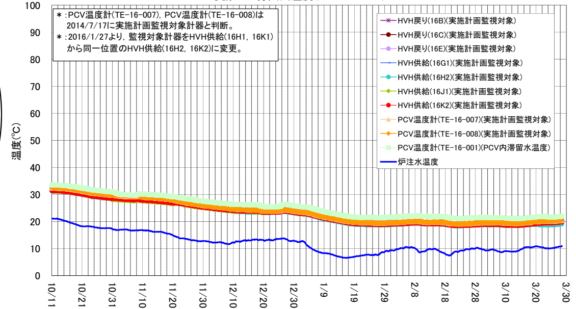
2号機 D/W雰囲気温度(10/11~3/28)
