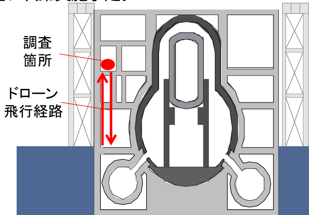
3号機原子炉建屋断面図
