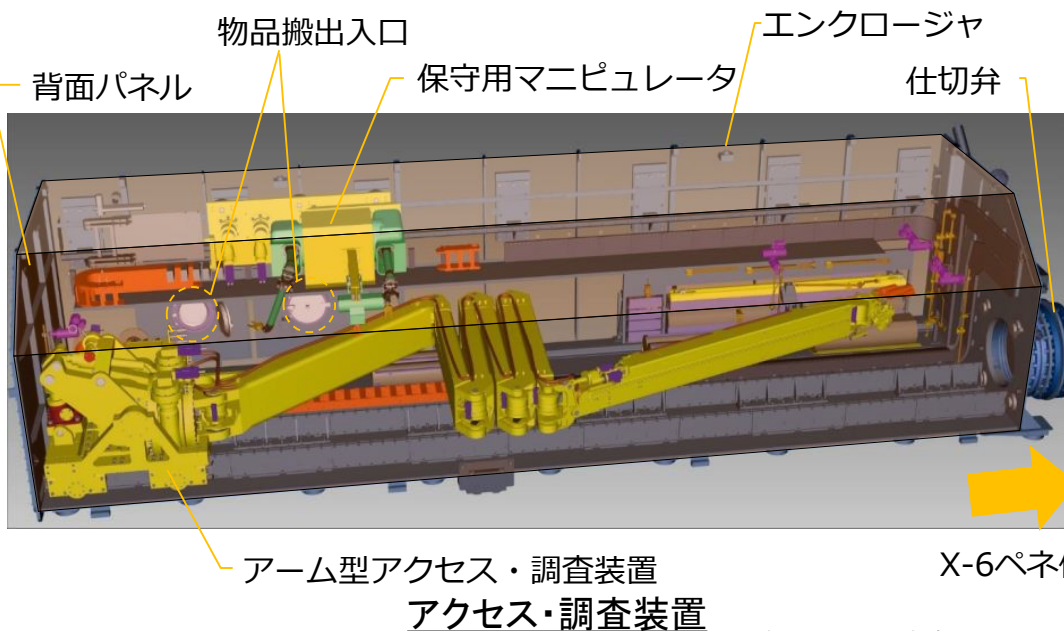
X-6ペネ前におけるアクセス・調査装置 設置案
