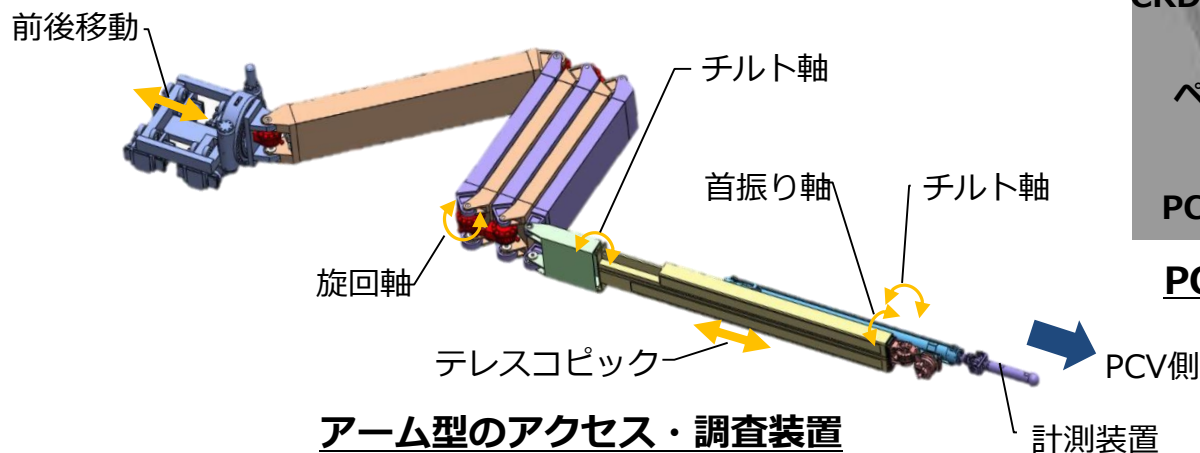
X-6ペネ前におけるアクセス・調査装置 設置案
