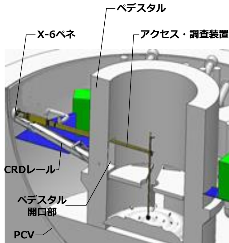
PCV内へのアクセス・調査装置の展開案
