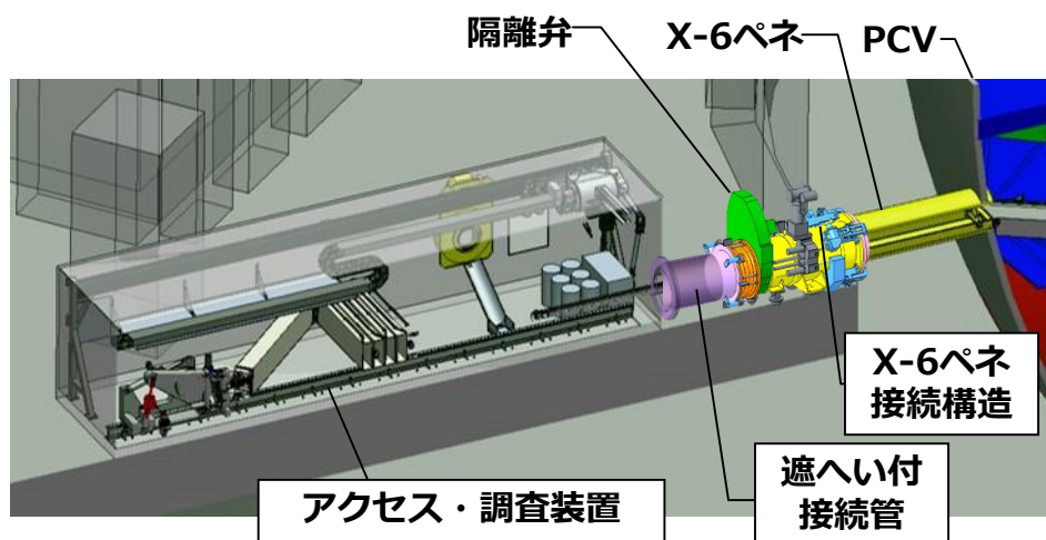
X-6ペネ前におけるアクセス・調査装置 設置案
