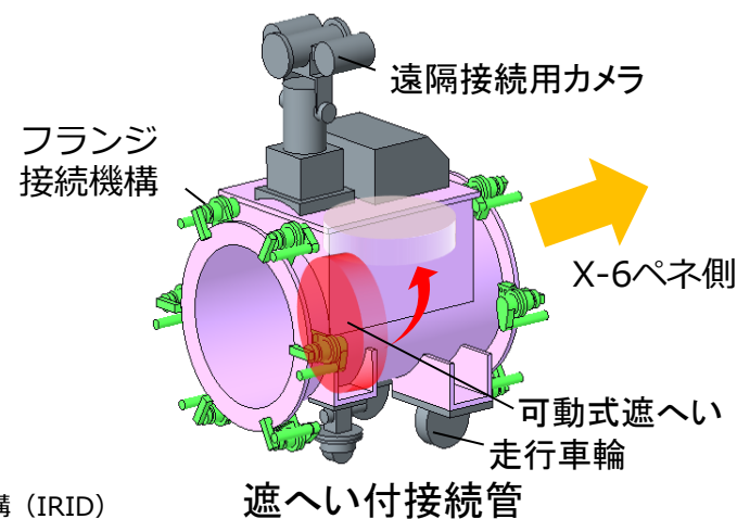
X6ペネ接続構造
