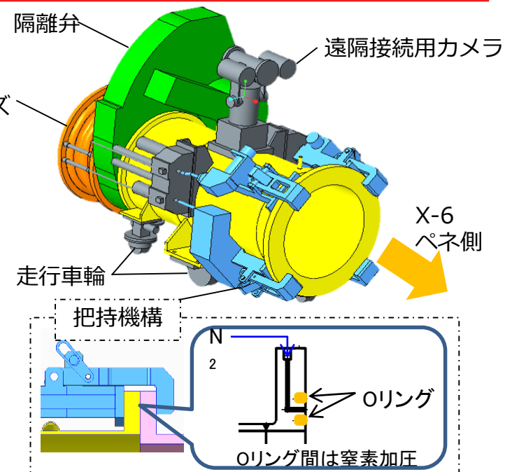
X6ペネ接続構造
