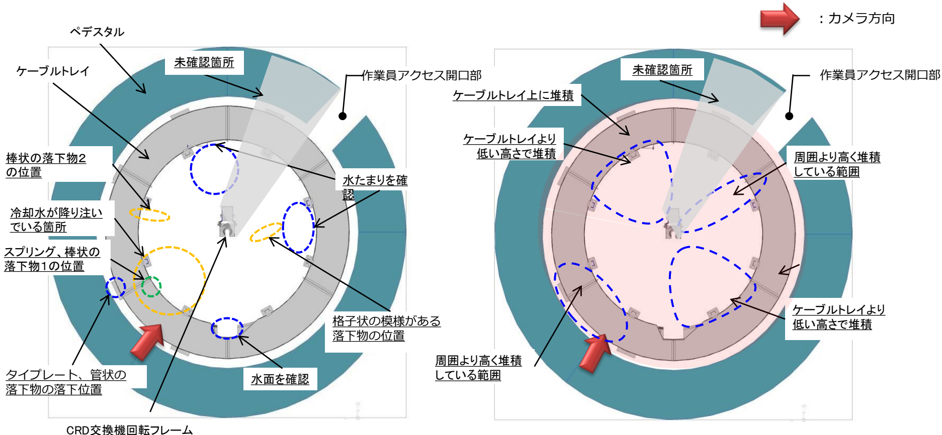
ペDESTAL底部の水たまり、落下物の確認状況
