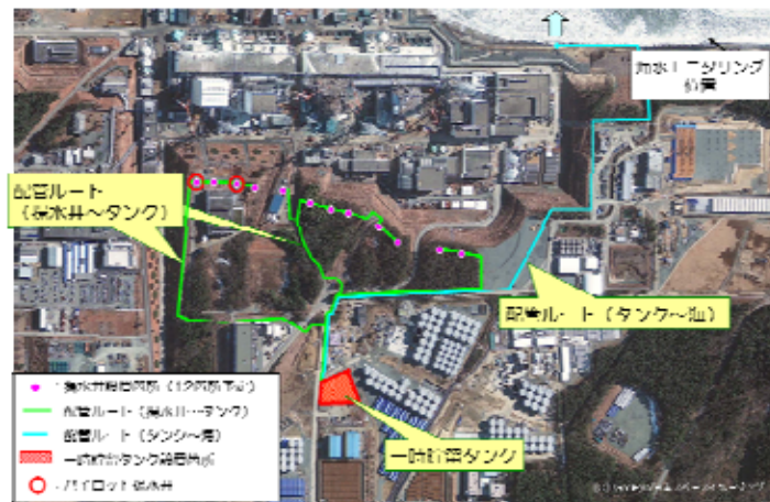
図 1：地下水バイパス設備概要
