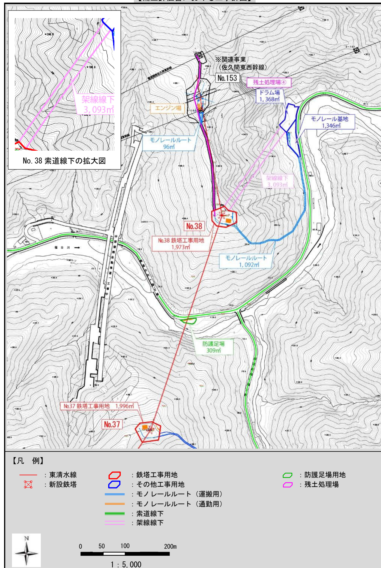
図 1.4.1-7(1) 工事計画詳細図 (No. 38 周辺)
