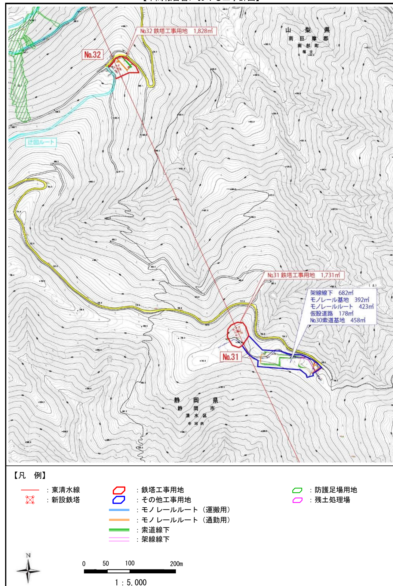
図 1.4.1-2(2) 工事計画詳細図 (No. 31 周辺)
