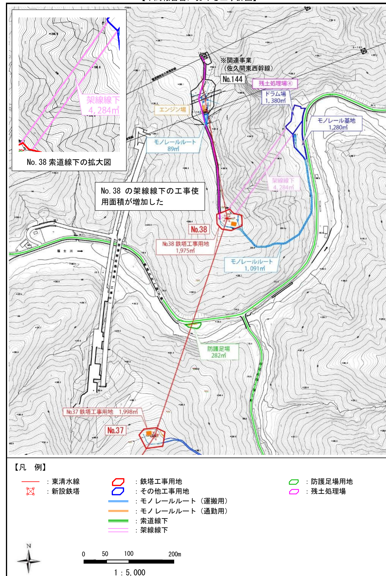
図 1.4.1-7(2) 工事計画詳細図 (No. 38 周辺)
