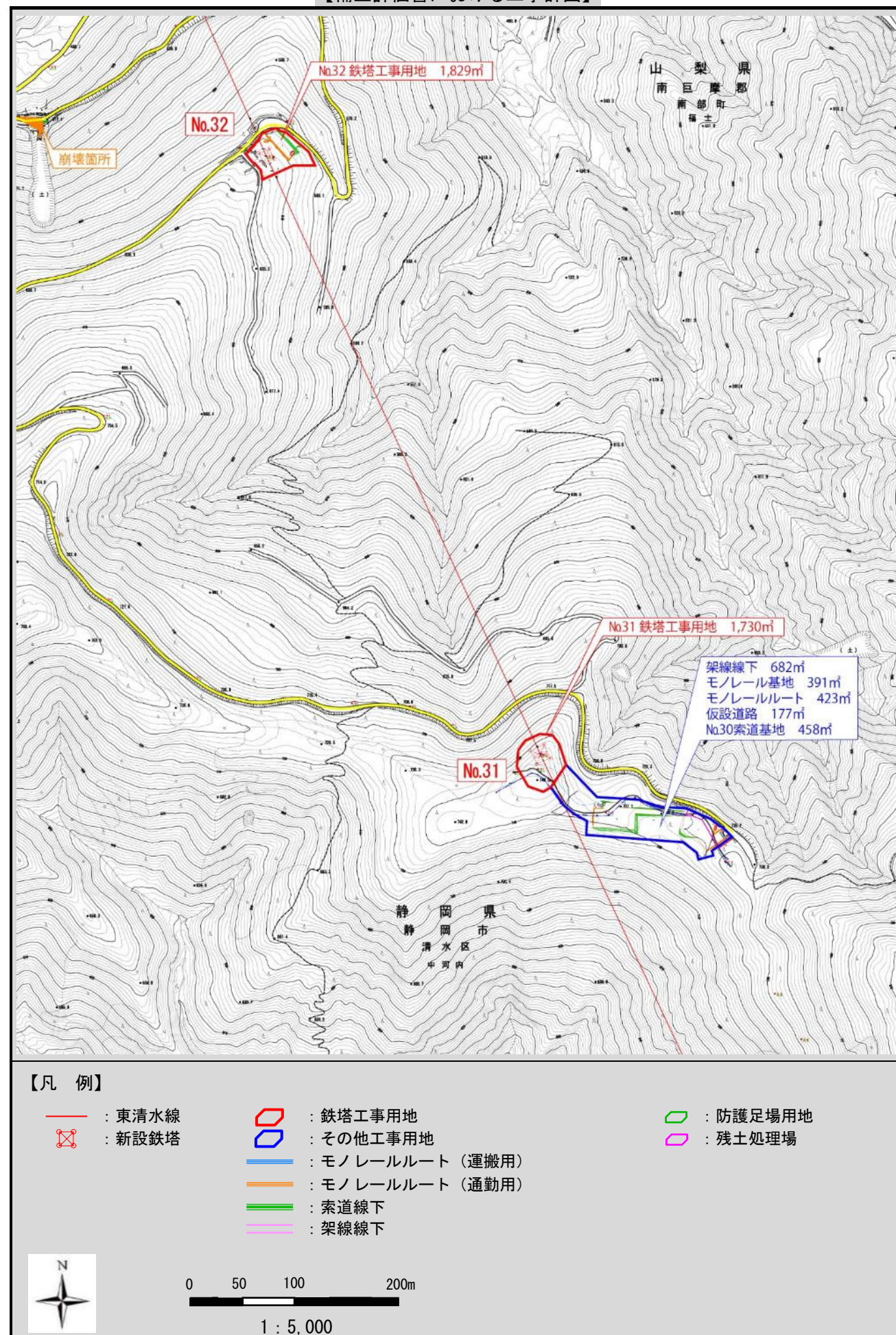
図 1.4.1-2(1) 工事計画詳細図 (No. 31 周辺)
