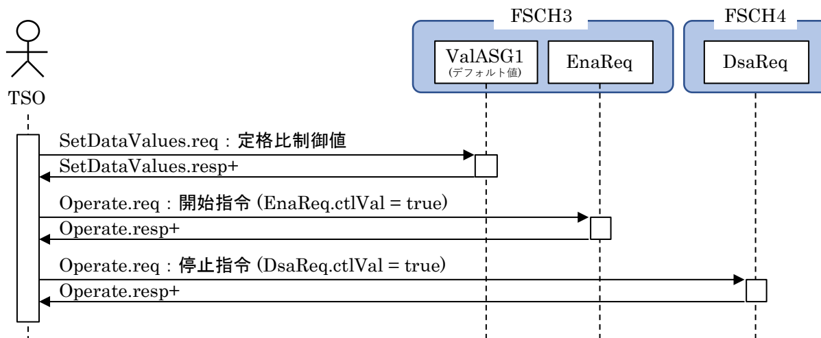
図9 デフォルト値の通信手順
