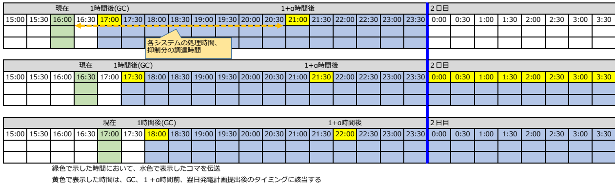
図2 各タイミングにおける制御値の更新範囲 (例：16:30 に翌日分の配信を開始する場合のイメージ)
