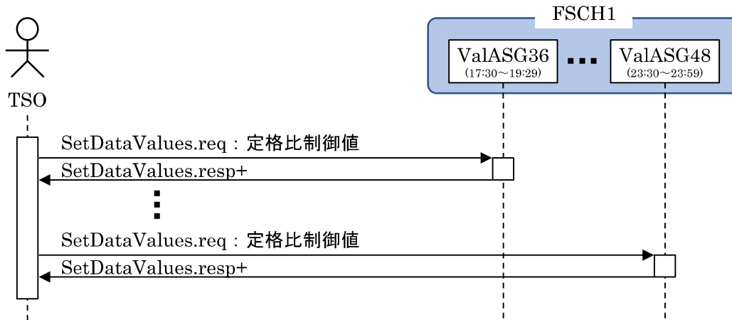
図8 16:30における当日残り分の制御値通信手順
