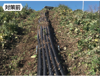
ケーブル盗難防止対策(タコムマット)施工例
