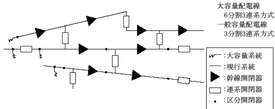
第Ⅲ－6図 架空配電系統の形態例
