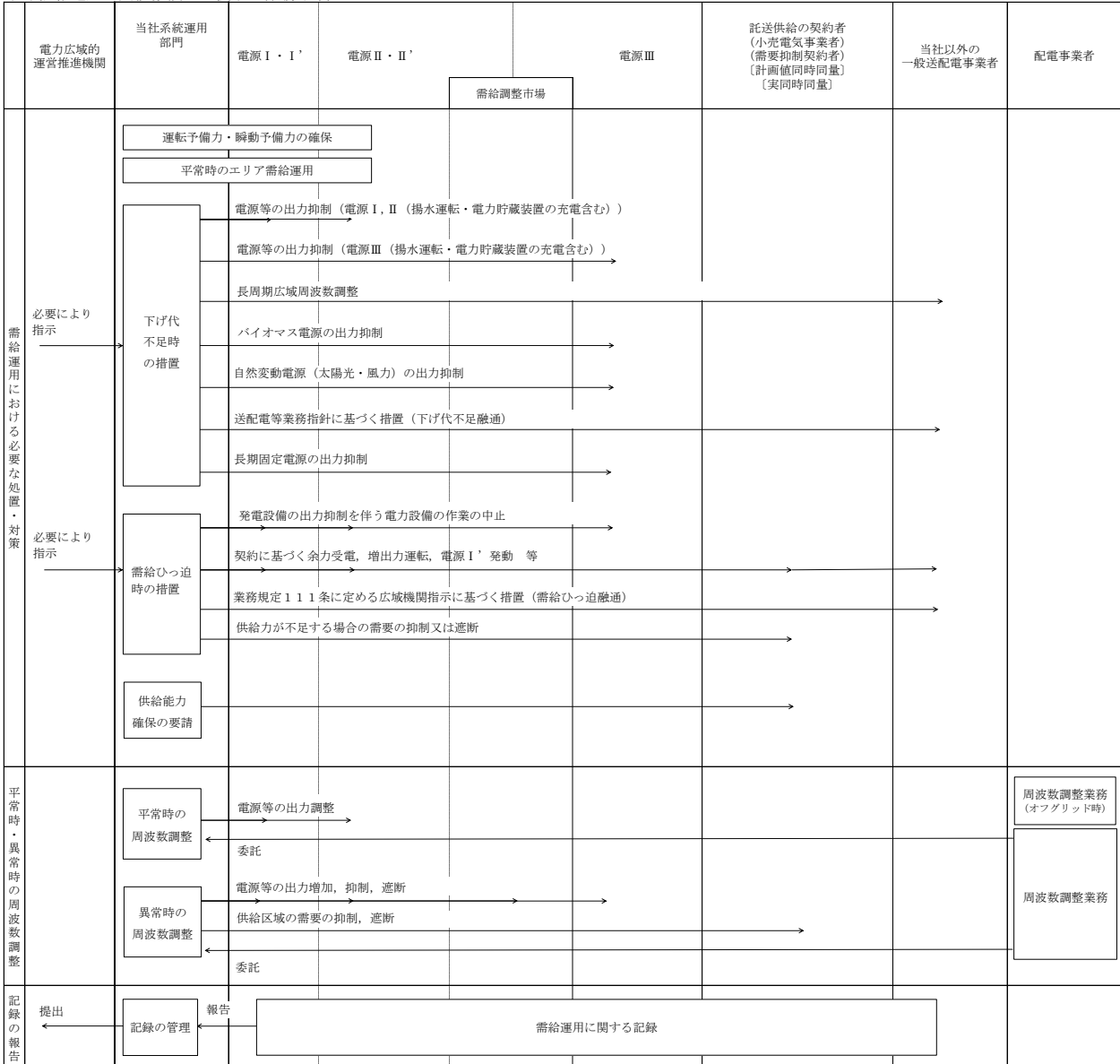
(2) 需給運用・周波数調整に関する業務手順
